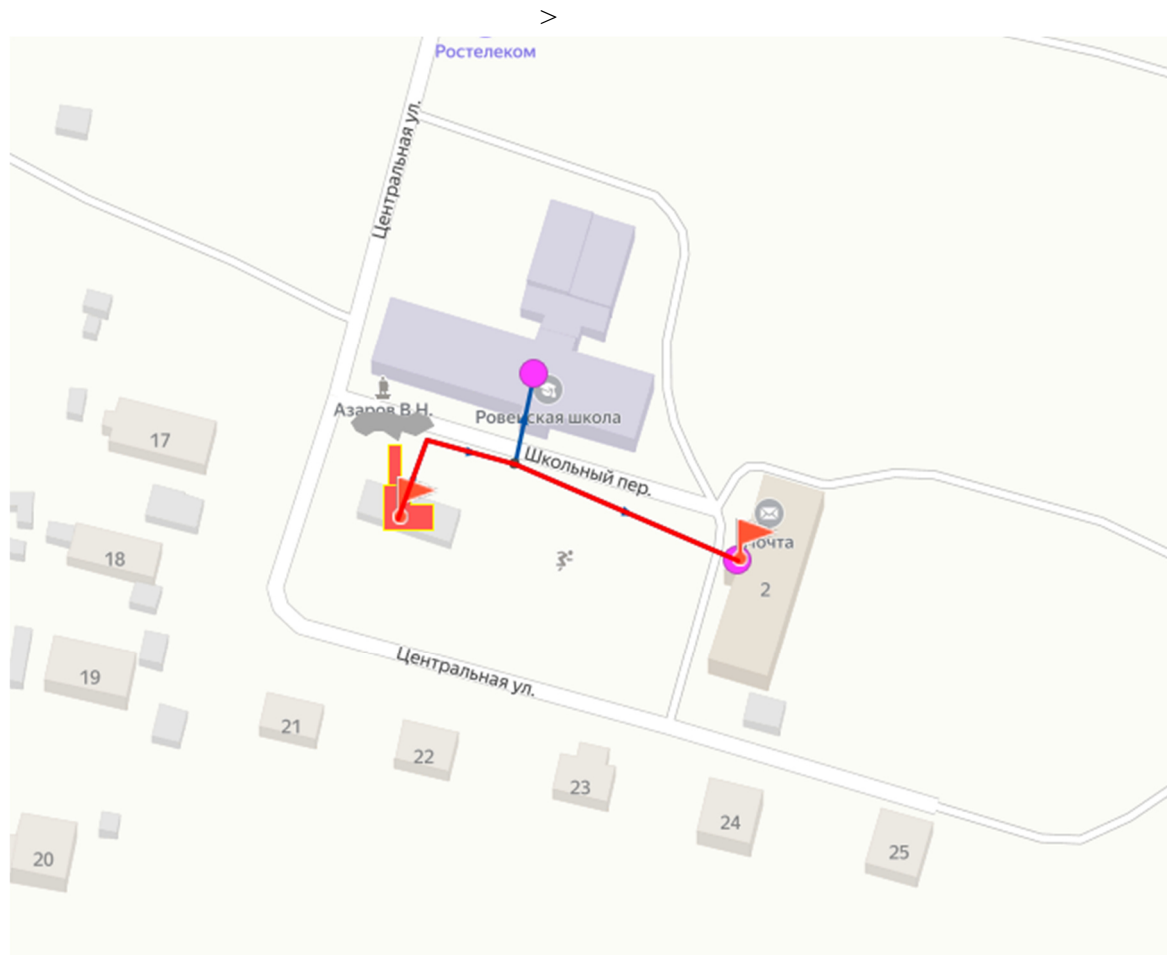
Рисунок 5 - Путь движения теплоносителя от источника тепловой энергии до конечного потребителя, в зоне действия котельной №10 н.п. Ровно
