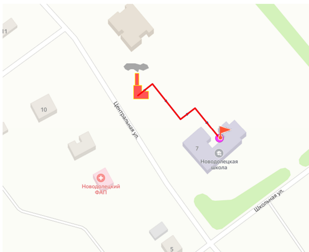
Рисунок 3 - Путь движения теплоносителя от источника тепловой энергии до конечного потребителя, в зоне действия ИТП №7 н.п. Н. Дольцы
